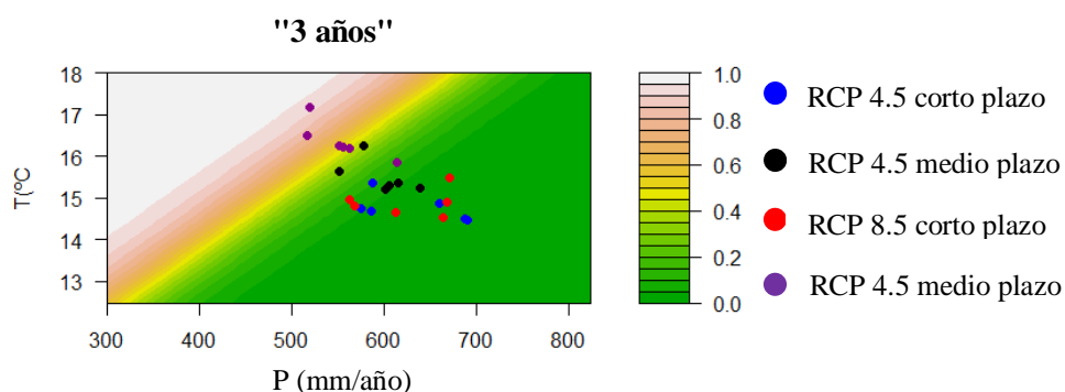
Figura 10.11. Mapa de curvas de nivel de probabilidad (modelo "3 años") y salidas de los modelos climáticos
