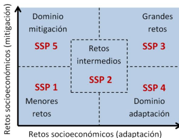
Figura 11.2. Desafíos mitigación/adaptación de los SSPs
